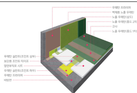
우레탄복합공사 상세
