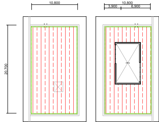
옥탑지붕층 평면도
